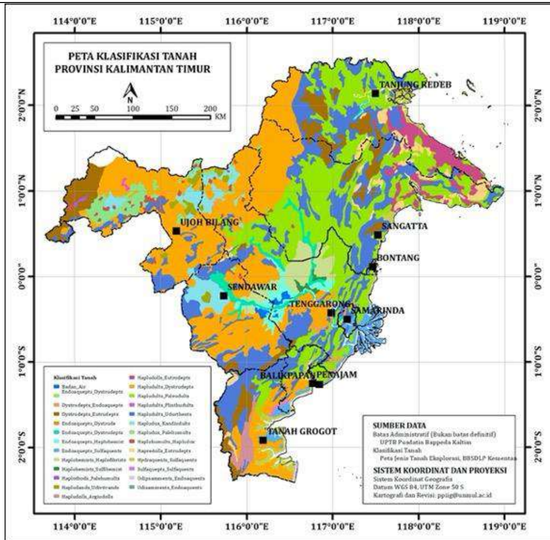
Gambar II - 1 Peta Klasifikasi Tanah Provinsi Kalimantan Timur
