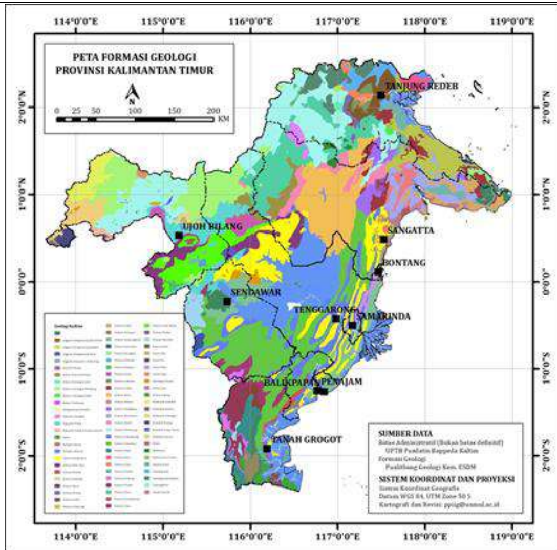
Gambar II- 2 Peta Formasi Geologi Provinsi Kalimantan Timur
